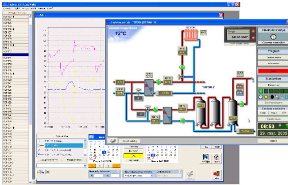
Figura 14: interfaccia SCADA per il monitoraggio e controllo sul desktop 10
